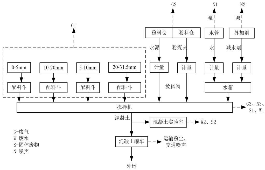
图 2-6 运营期工艺流程图
