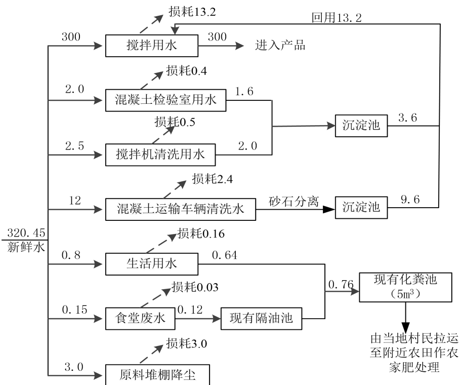
图 2-5 本项目验收阶段水平衡图 单位：m 3 /d
